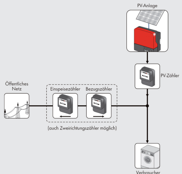
Abb. 4: Zählerkonfiguration zur Eigenverbrauchsmessung
